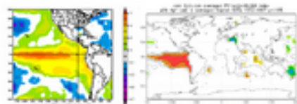
Fig. 4 Correlaciones entre la temperatura del Mar Pacífico y las precipitaciones en la IV Región (a) y el caudal en el Río Elqui (b)
